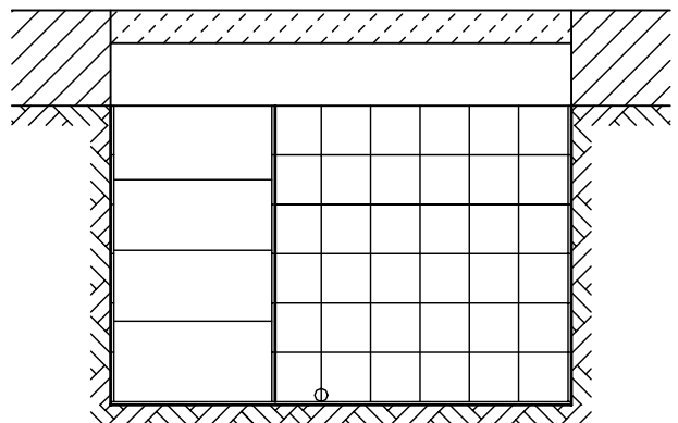
Schnitt C-C
