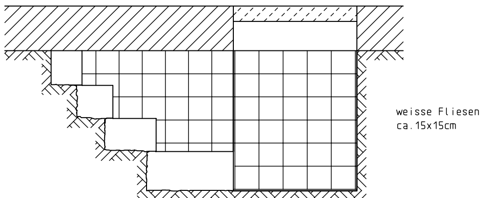
Schnitt A-A
