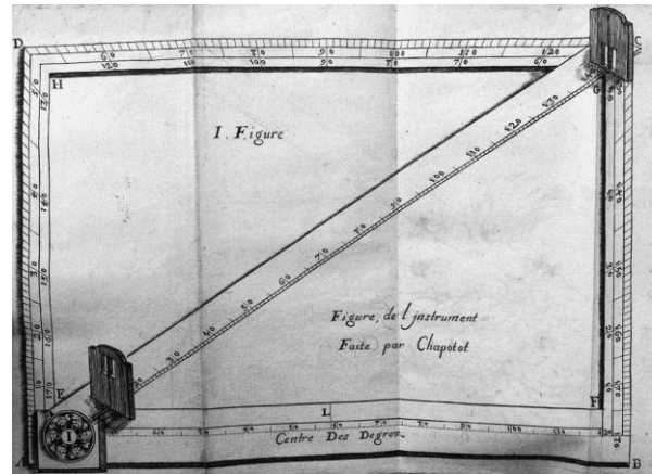
Abbildung 6.2: Zeichnung eines Universalinstruments zur Vermessung vom französischen Mathematiker Jacques Ozanam (1640-1718). Aus >L'usage de l'Instrument universel<, 1688, Paris. Digitalisiert: MDZ https://tinyurl.com/jmtbyken .
