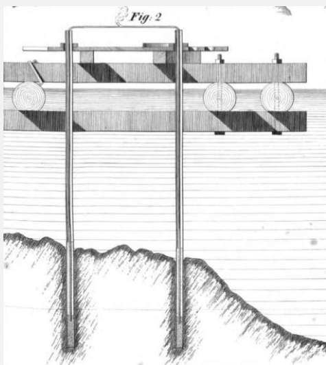
Abbildung 10.11: Floss zum Bohren von Sprenglöchern in den Quarzit des Binger Lochs und zum Einbringen der >Pulverbüchsen<. Quelle: von Bergh, Felsensprengungen im Rhein bei Bingen, 1834.
