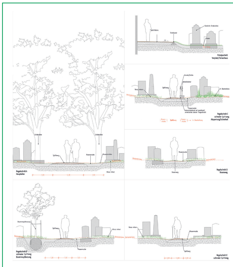
Abb. 3 Jüdischer Friedhof Währing, Entwürfe zur Weggestaltung, Landschaftsarchitekt Gerhard Rennhofer
